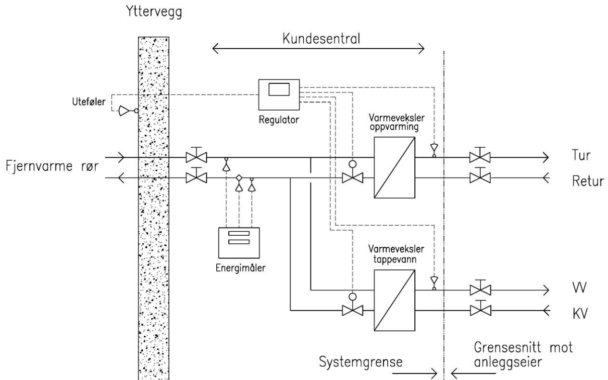
Figur 4-1 Grensesnitt mellom VV og anleggseier
